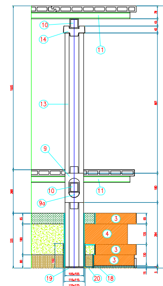
PARTICOLARE COLONNE
