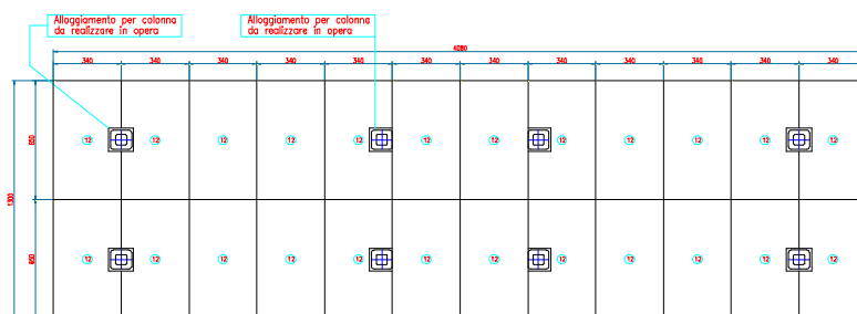
SEZ. B-B
